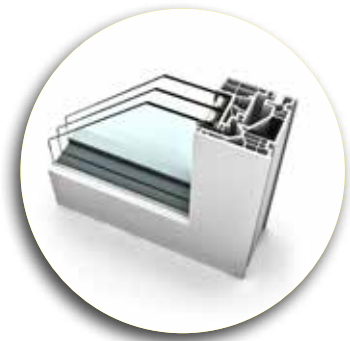
Kunststoffausführung (aussen)
