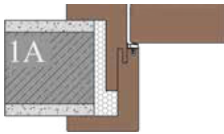
Zargensystem (1A) INTRA 63-75 TS40 Wandüberstehendes Zargensystem 2-schalige Zarge auf der Wand Spiegelbreite 63mm / 75mm
